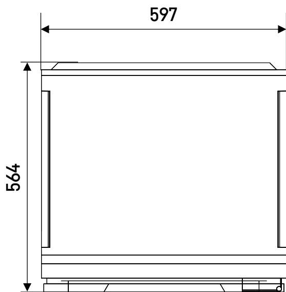
製品本体寸法（天面図）
