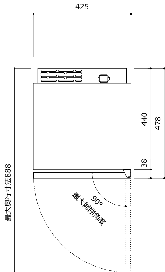
平面図
