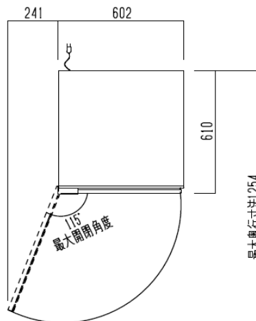
平面図
