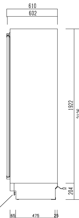
側面図
