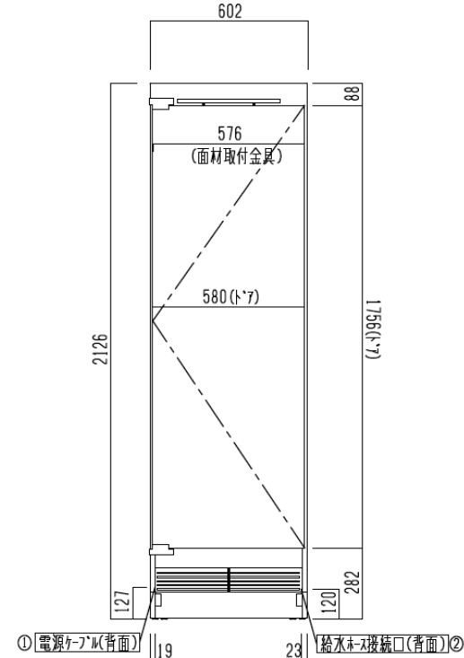
正面図
